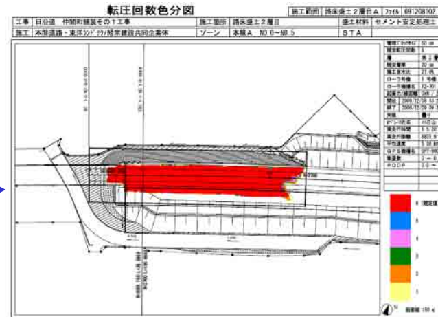
品質管理帳票: 転圧回数色分図
