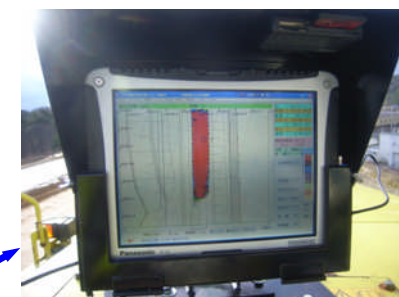
転圧回数確認モニター
