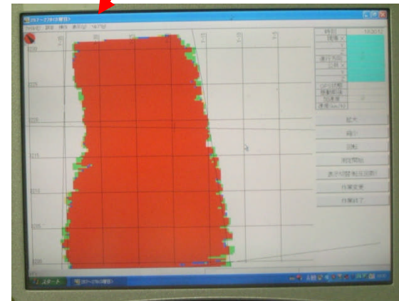
車載モニターにてリアルタイムに 転圧面の確認
