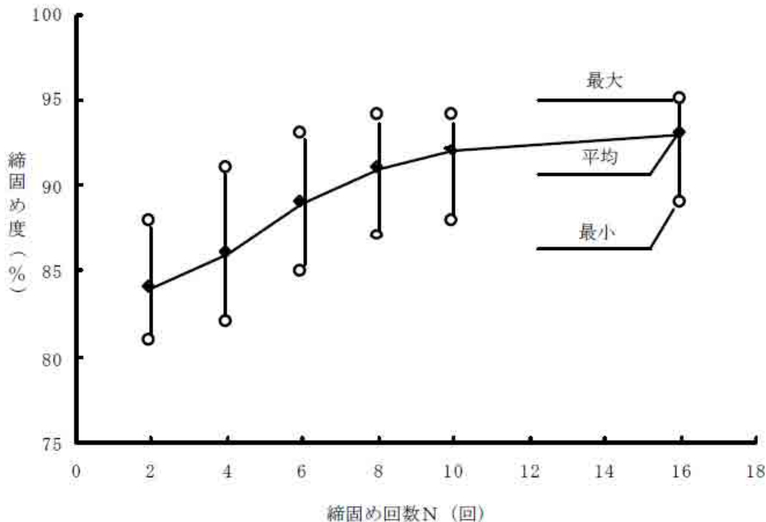
試験施工結果の作図例(締固め度で管理できる材料:RI計による測定例)
