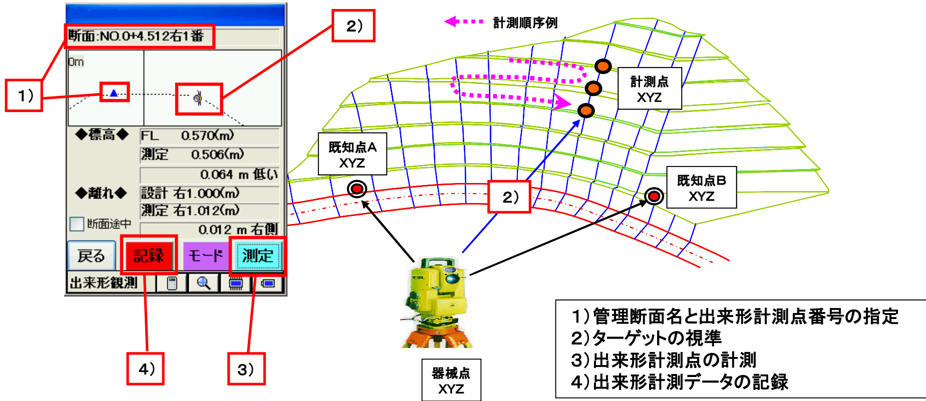
図1-10 現場における作業手順例
