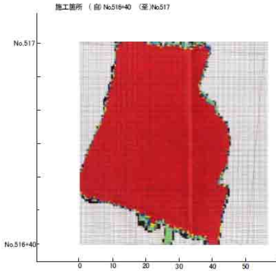
締固め回数分布図例
