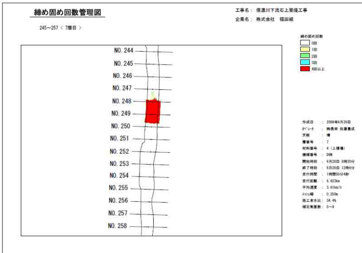
締固め回数分布図
